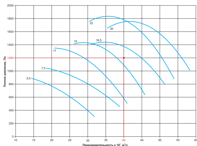
Аэродинамические характеристики РОСА-500-7,1
