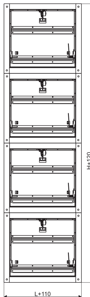
5и - четыре кассеты по H (4 привода)
